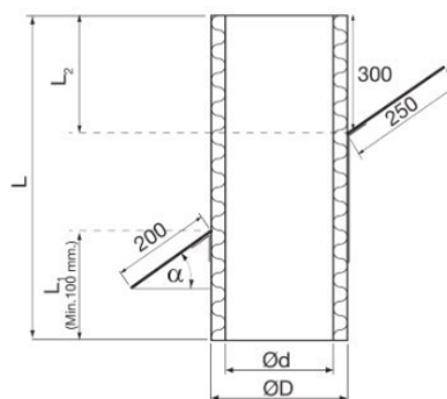
Isoleret taggennemføring
