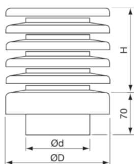
Indtagshætte
