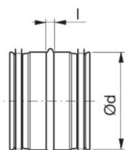
Nippel
