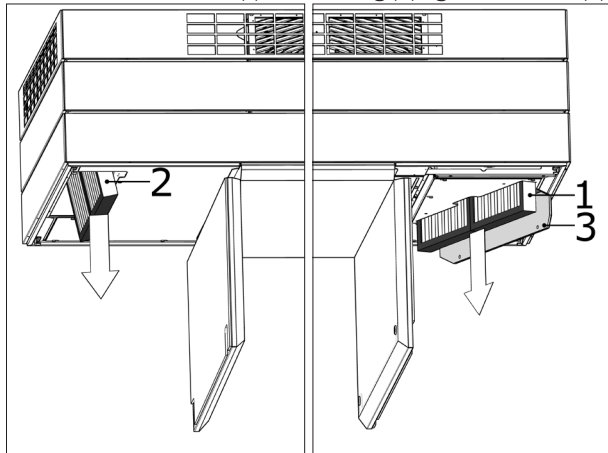
AM1000: Tilluftsfilter (1) under et låg (3) og fraluftsfilter (2).
