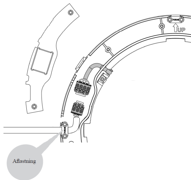
Figur 39 - Kabeltilgang fra venstre med aflastning i Klemrække 3
