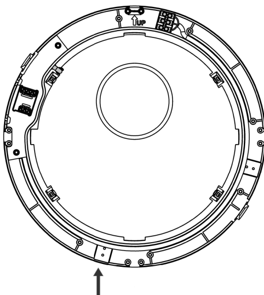
Figur 36 - Placering af Klemrække 2 ved kabeltilgang nedefra
