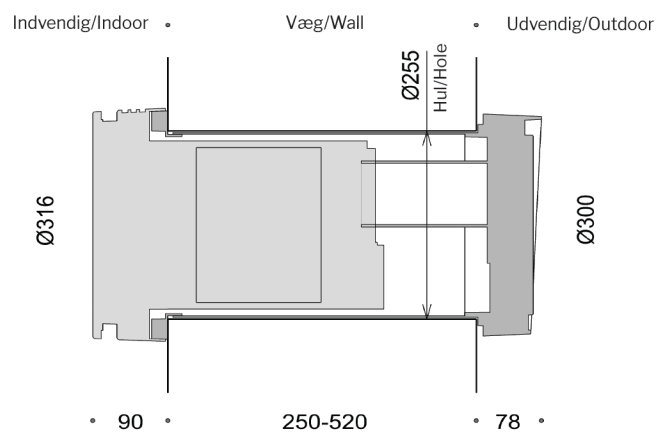
Figur 2 - Dimensioner. Alle mål i [mm]
