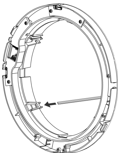
Figur 20 – Kabelbinderne fra den udvendige hætte føres ind i det indvendige vægdæksel
