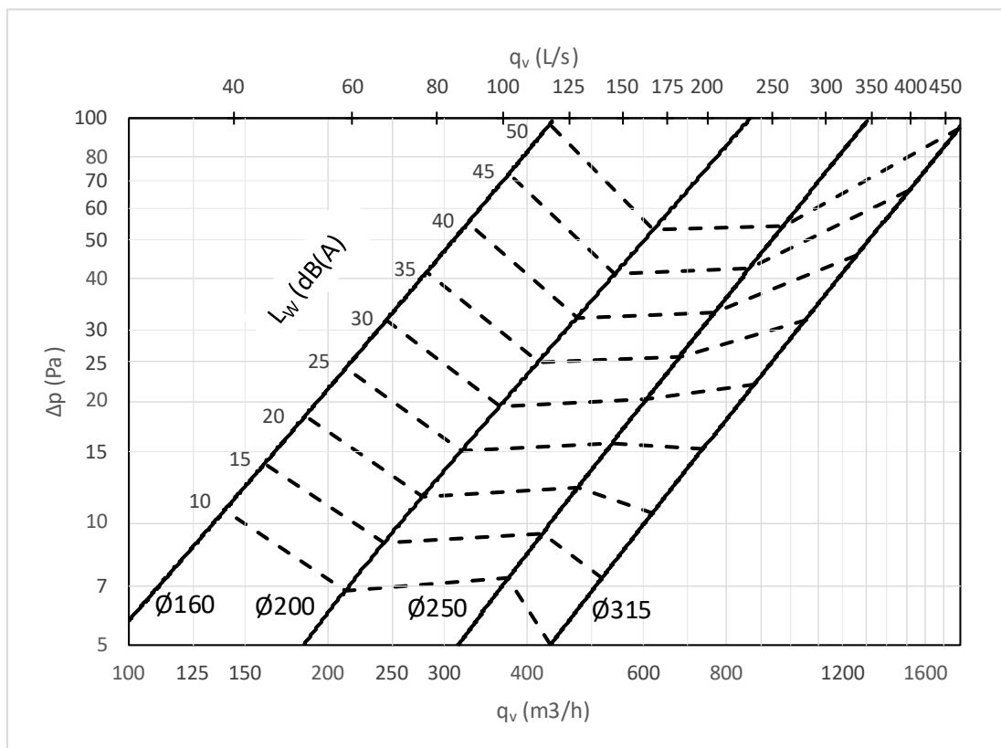
Figur 1 - Luftmængde q_v [l/s]; [m 3 /h], tryktab \Delta p [Pa] og lyd effektniveau LWA [dB(A)] vises i grafen.
