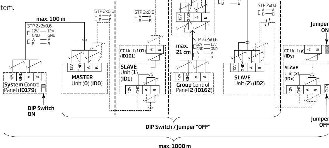
Eksempel el-diagram dataledninger:
