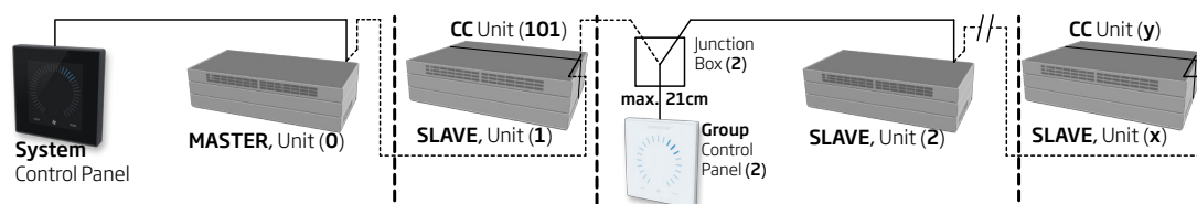
Eksempel el-diagram dataledninger:
